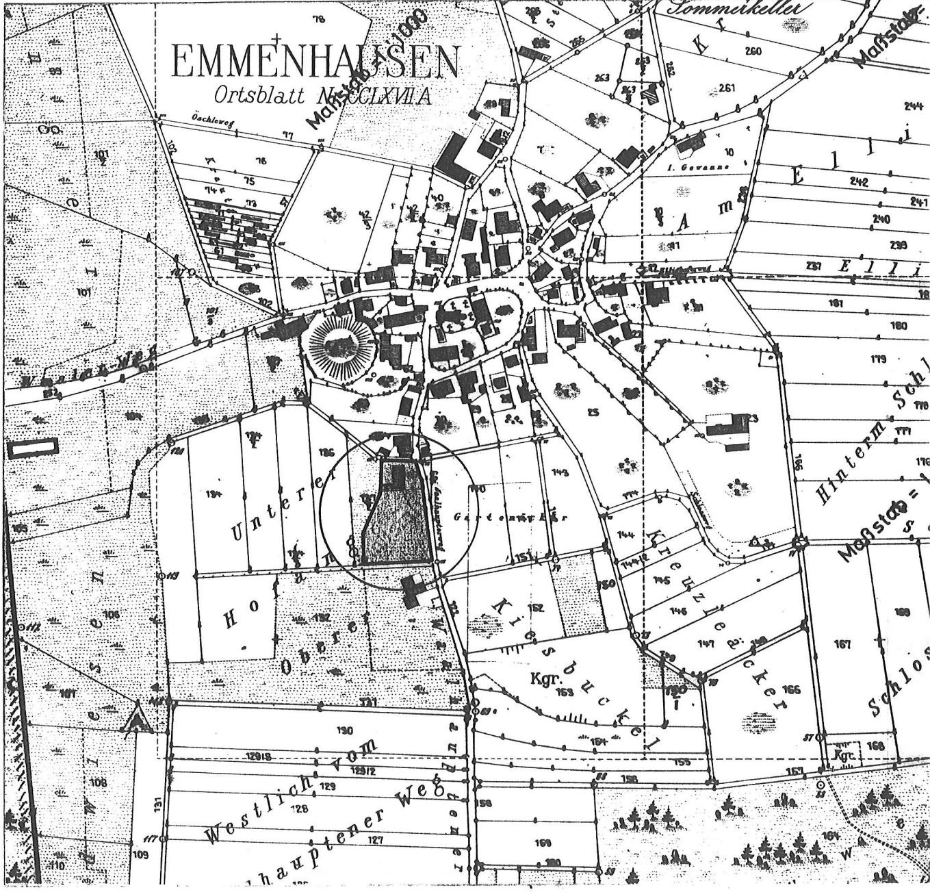
ÜBERSICHTSPLAN M 1:5000
